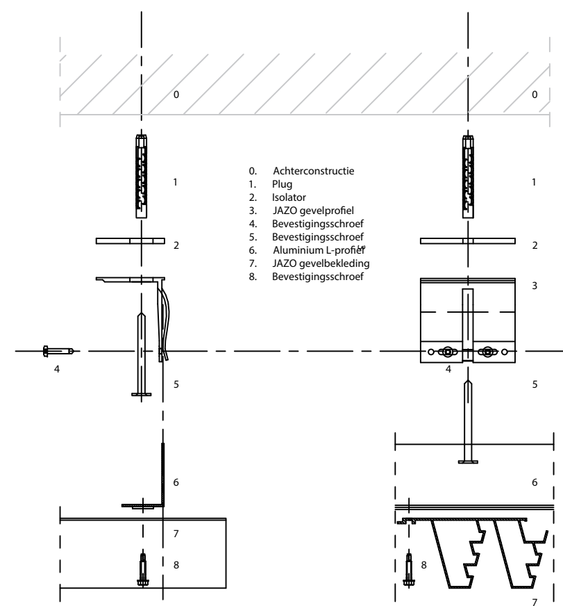
Horizontale doorsnede
